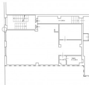
PIANTA PIANO PRIMO scala 1:100
